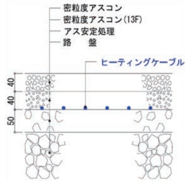
車道/アスファルト舗装
