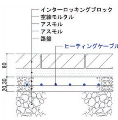
歩道/インターロッキング
