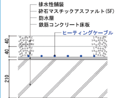
車道/橋梁舗装
