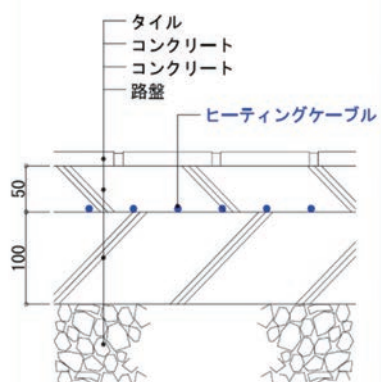
歩道/タイル仕上げ
