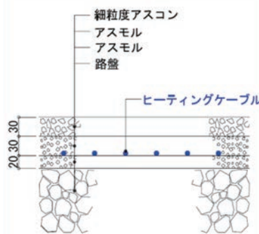
歩道/アスファルト舗装
