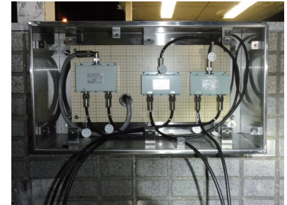
施工例 (屋外無線機接続端子箱内)
